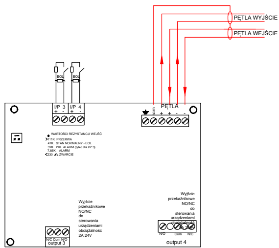
Schemat połączeń modułu /2IO
